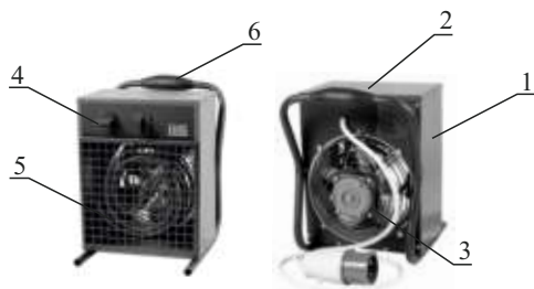
рис.1 Тепловентилятор
