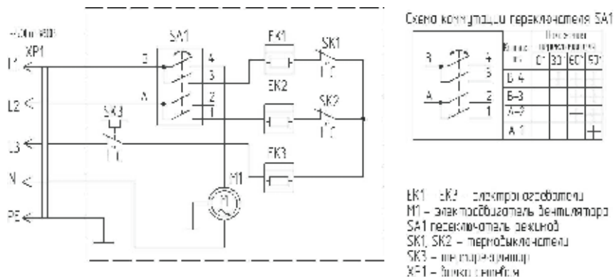
Рис. 4 Схема электрическая тепловентилятора ТВ 5/7 (380 В)
